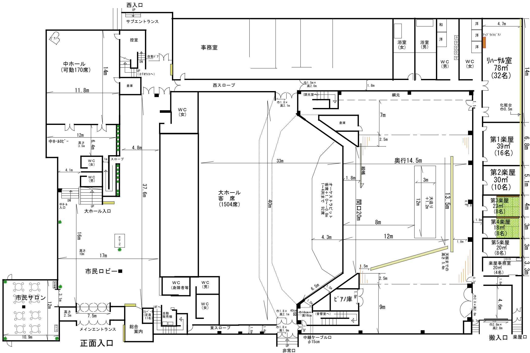
上越文化会館1F平面図
